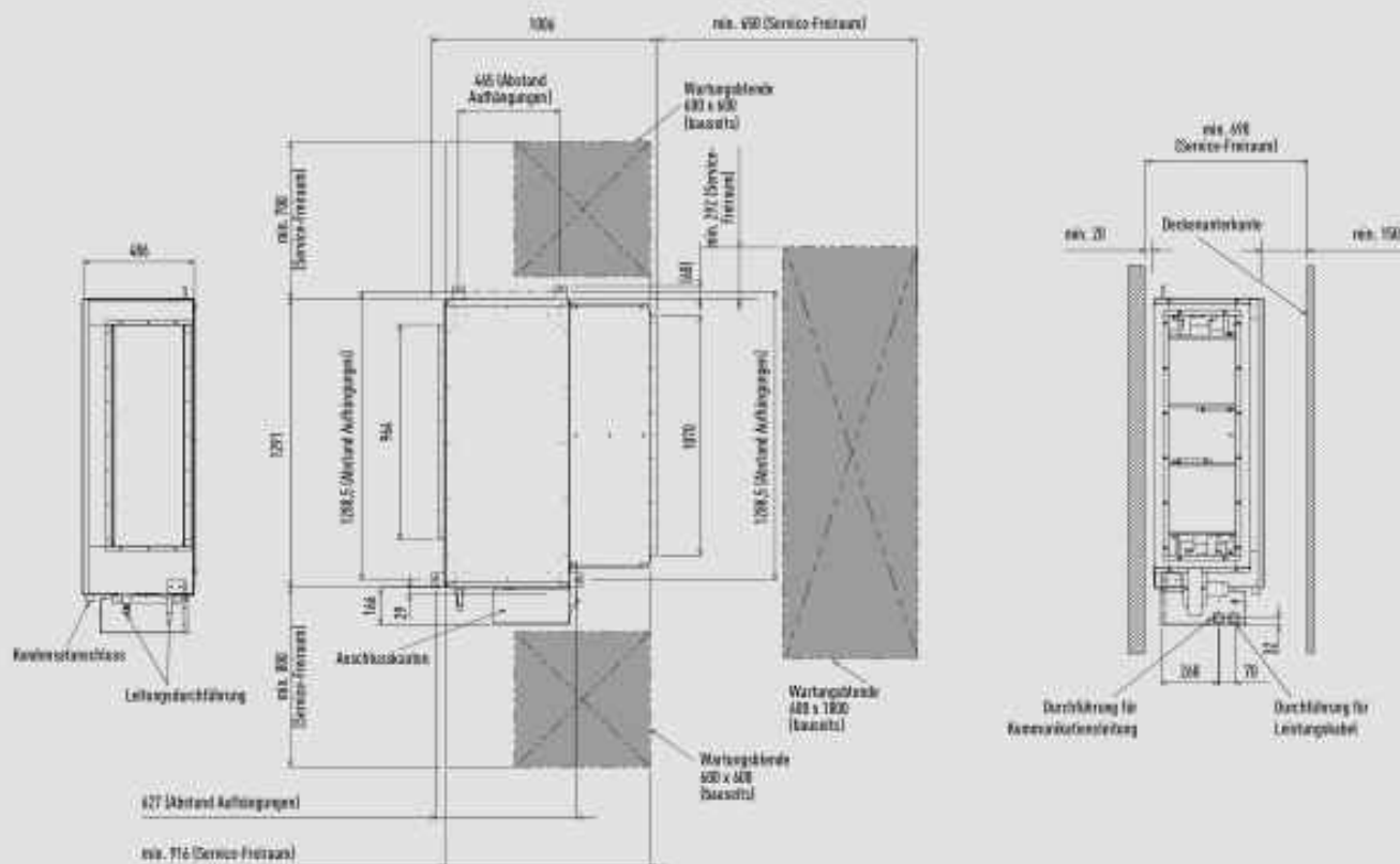
Abmessungen der Aufhängungsabstände und des Geräts sowie des mindestens erforderlichen Service-Freiraums.
