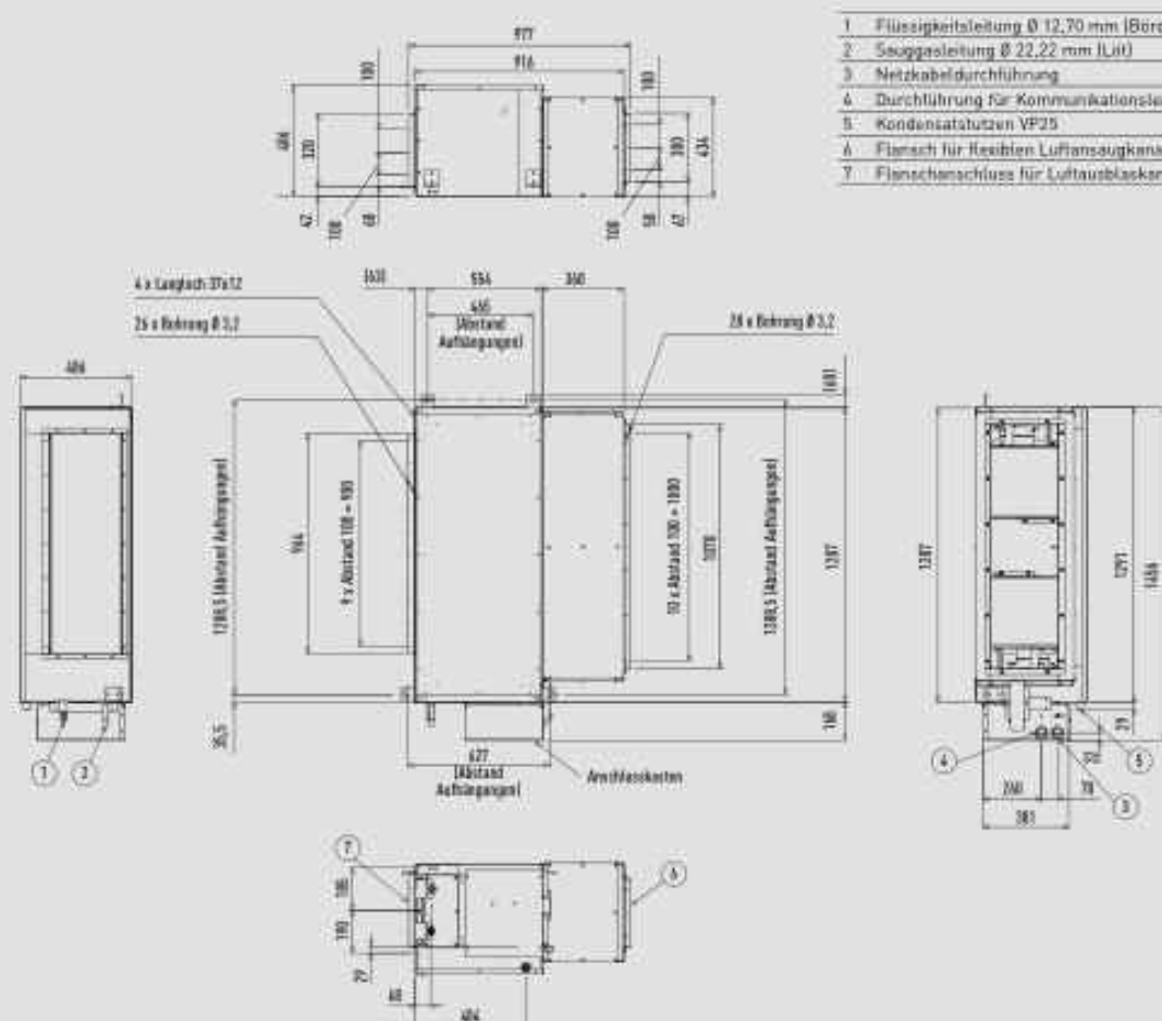
Abmessungen der Aufhängungsabstände und des Geräts sowie des mindestens erforderlichen Service-Freiraums.
